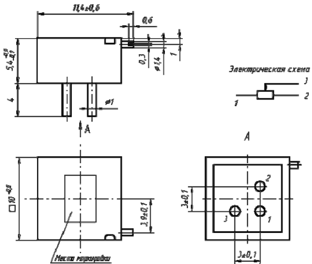
Резистор типа СП5-2ВБ
