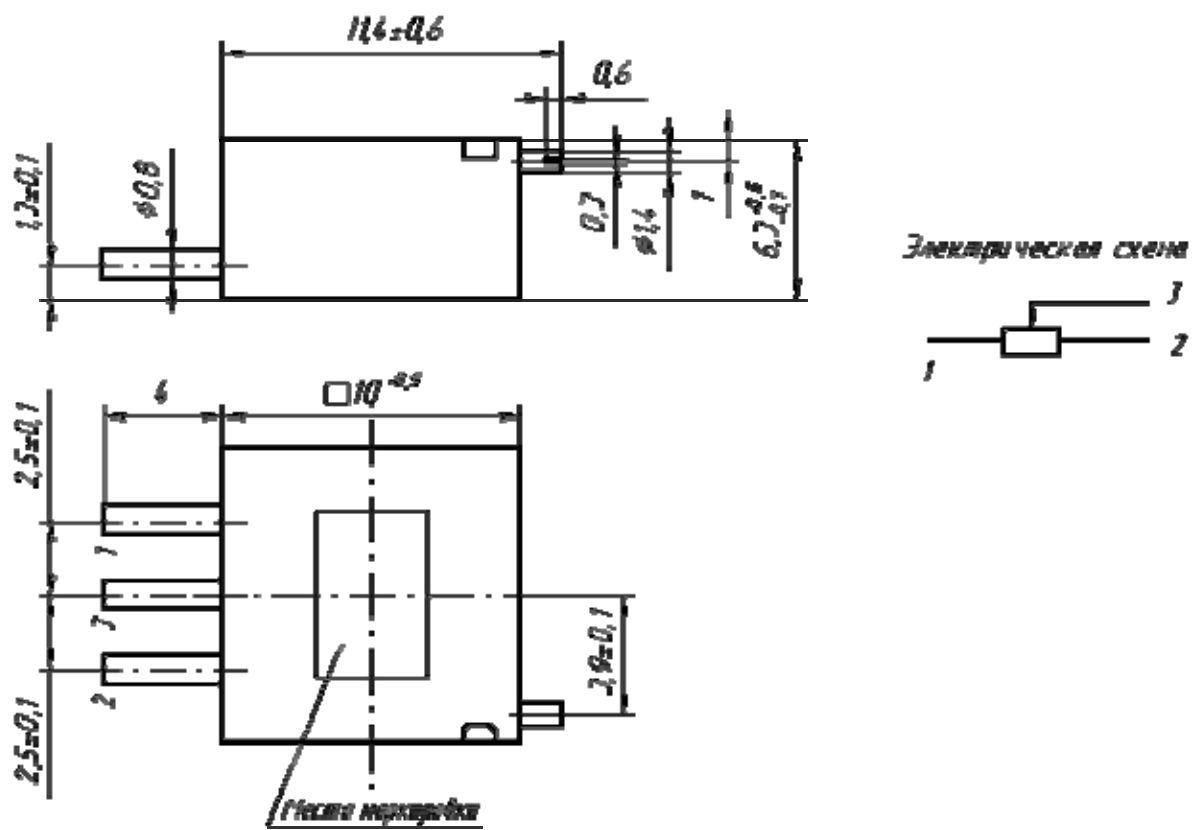
Резистор типа СП5-2ВБ
